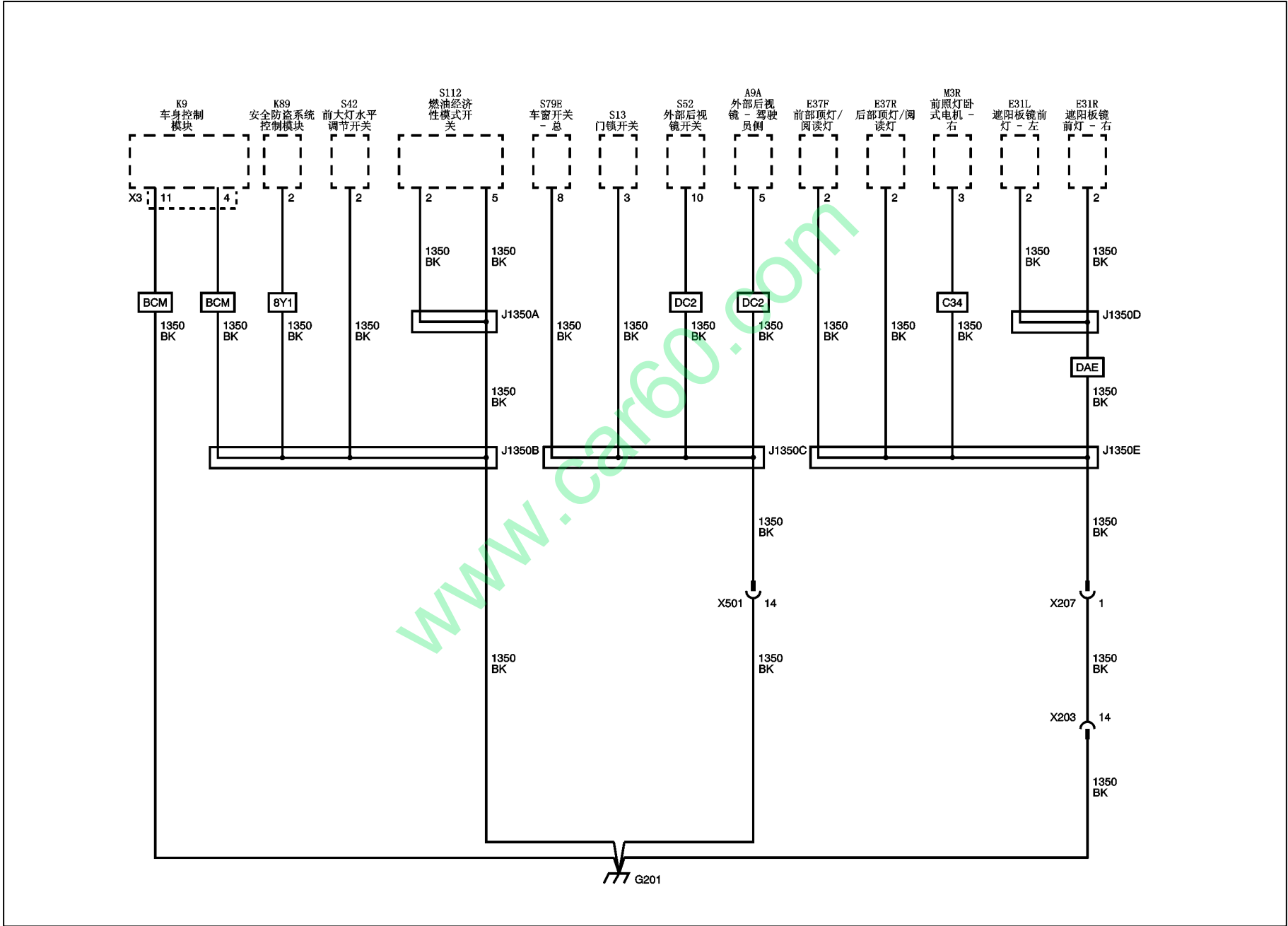
搭铁示意图 (G201 搭铁)
