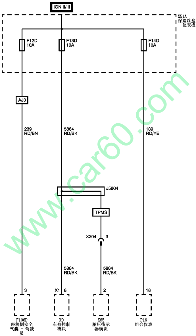
电源分布示意图 (F12D, F13D, F14D 保险丝)
