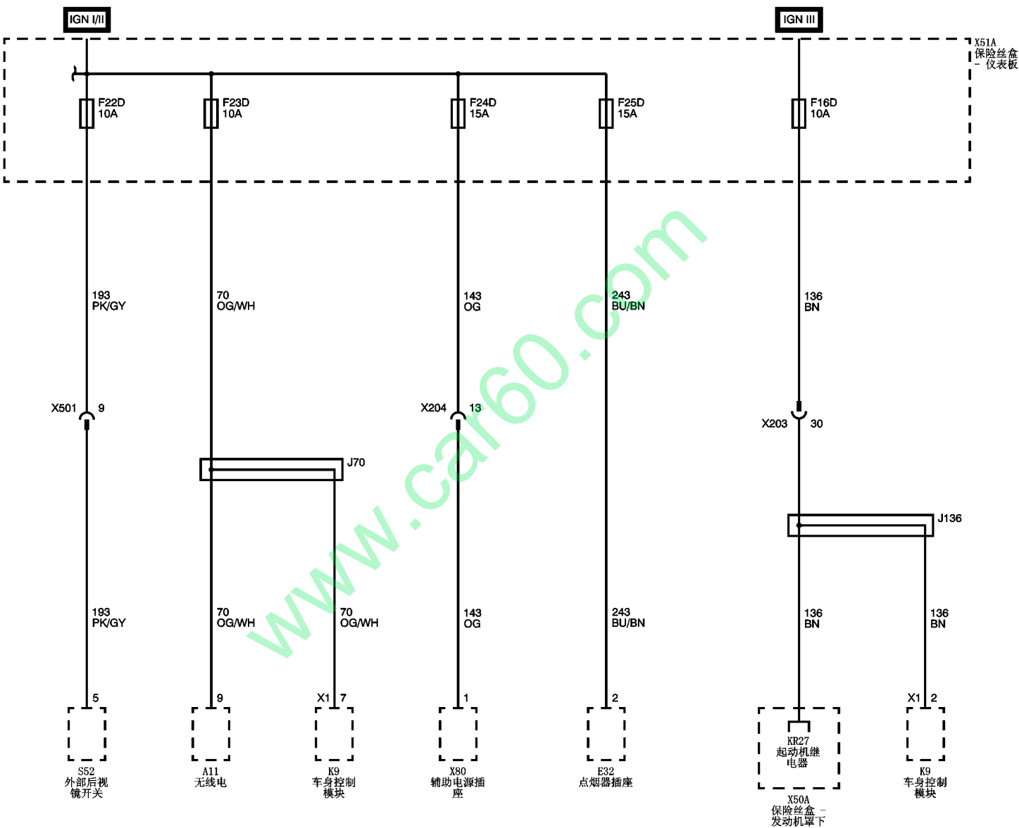
电源分布示意图 (F16D, F22D, F23D, F24D, F25D 保险丝)
