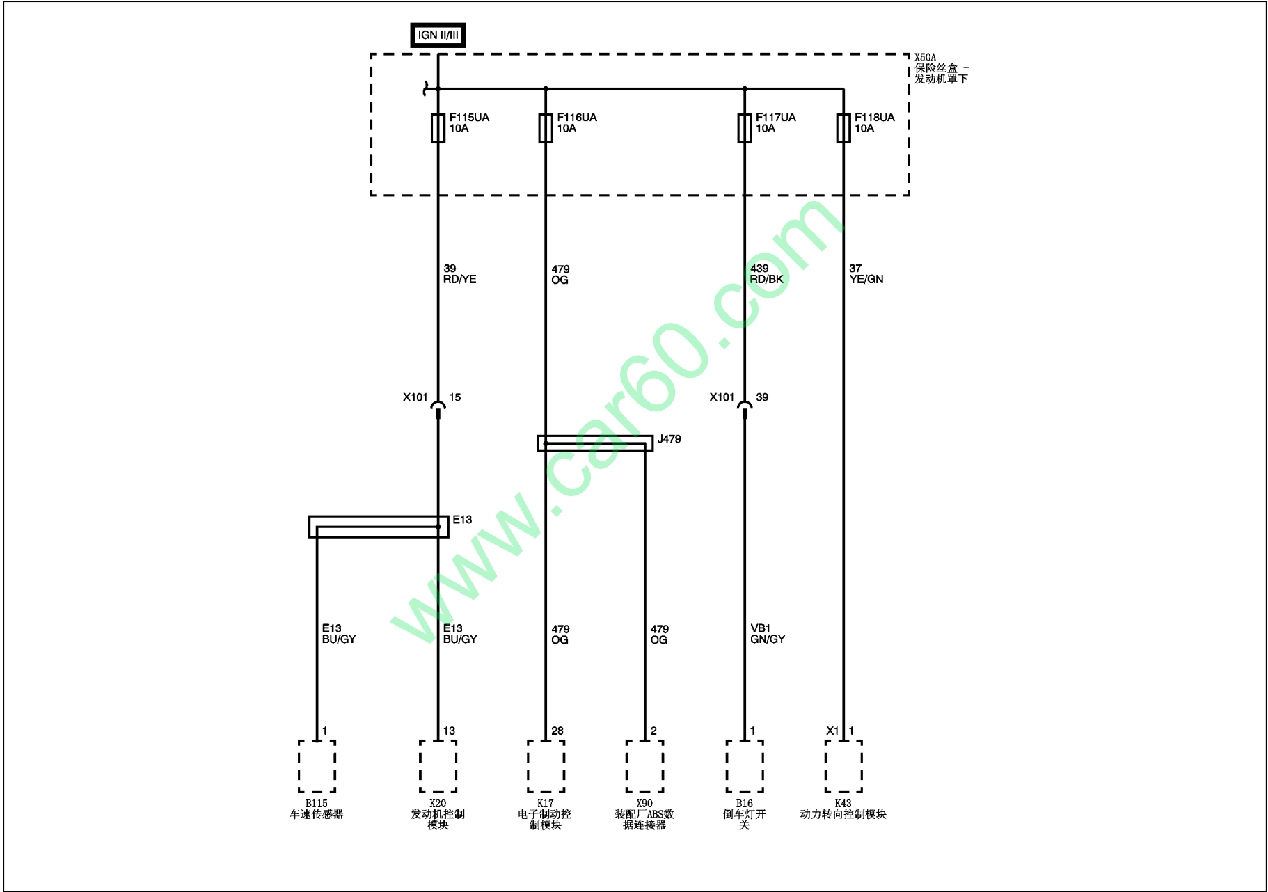
电源分布示意图 (F115UA, F116UA, F117UA, F118UA 保险丝)
