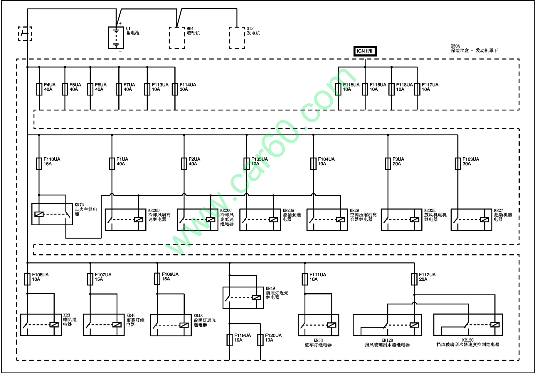
前舱保险盒电源分布
