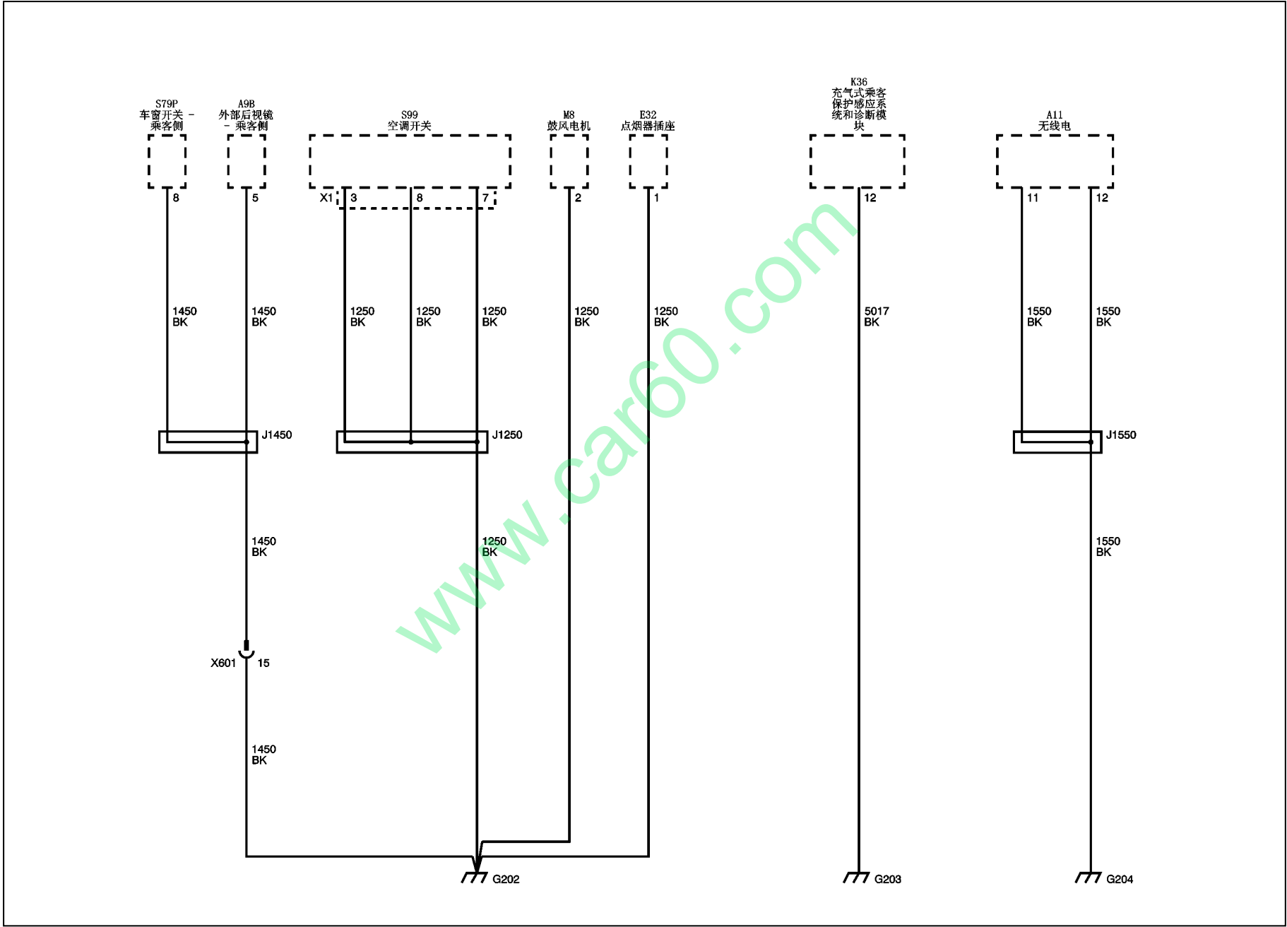
搭铁示意图 (G202, G203, G204 搭铁)
