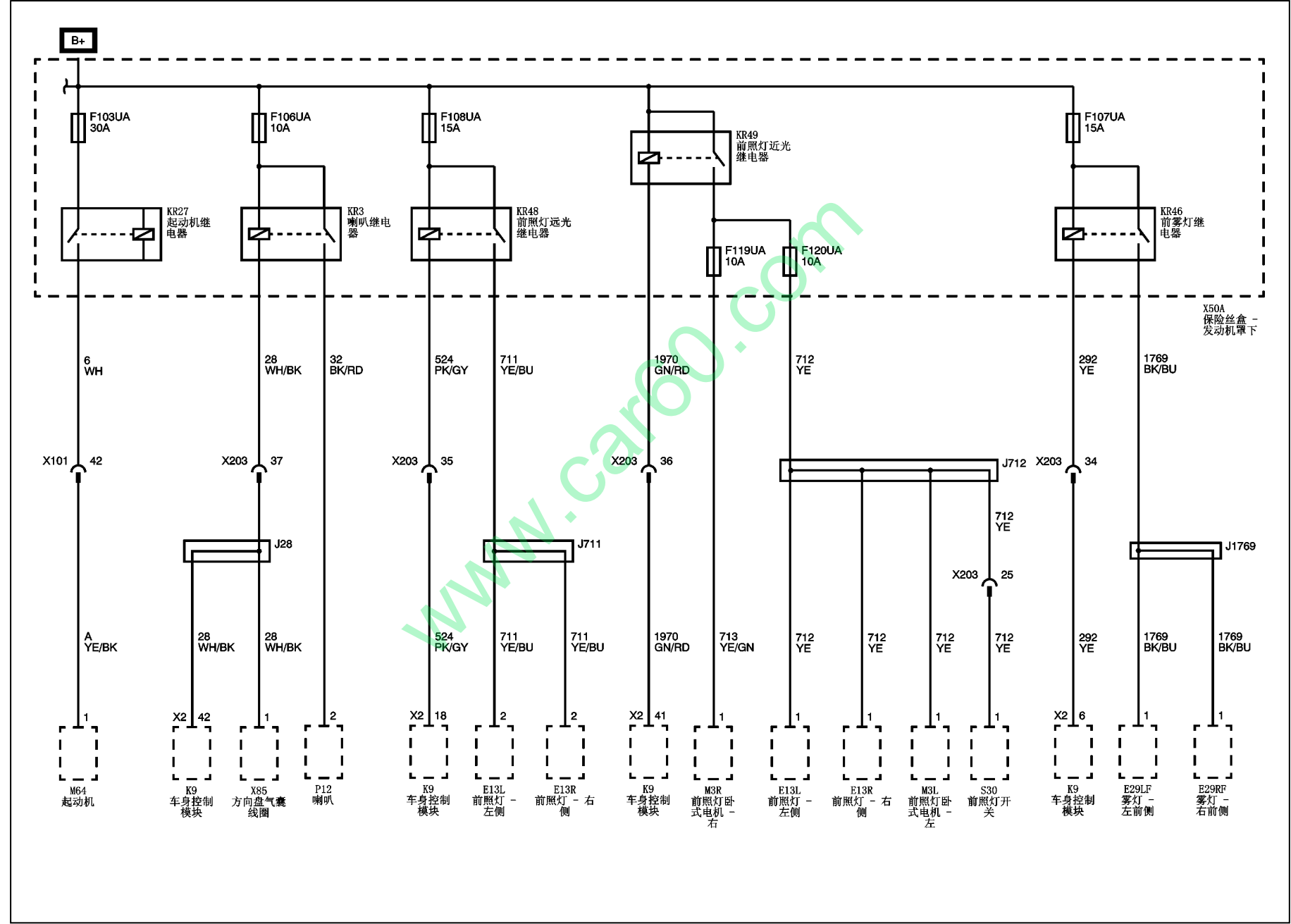
电源分布示意图 (F103UA, F106UA, F107UA, F108UA, F119UA, F120UA 保险丝)
