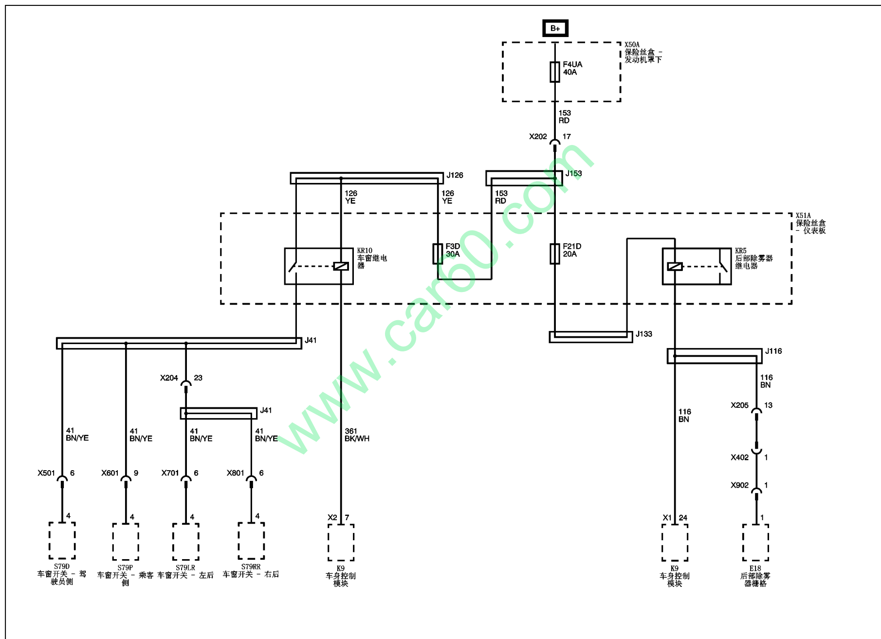
电源分布示意图 (F4UA, F3D, F21D 保险丝)
