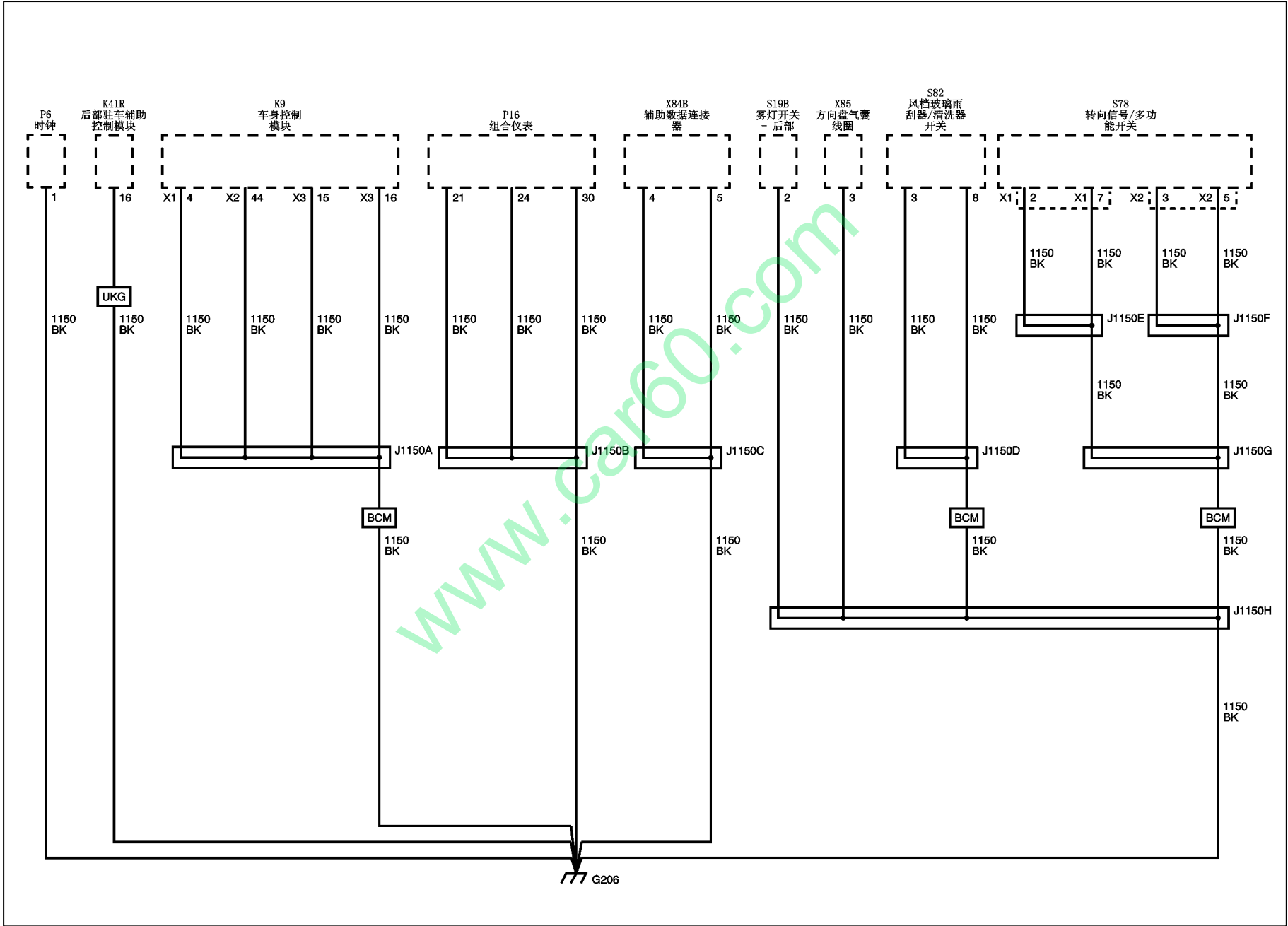
搭铁示意图 (G206 搭铁)
