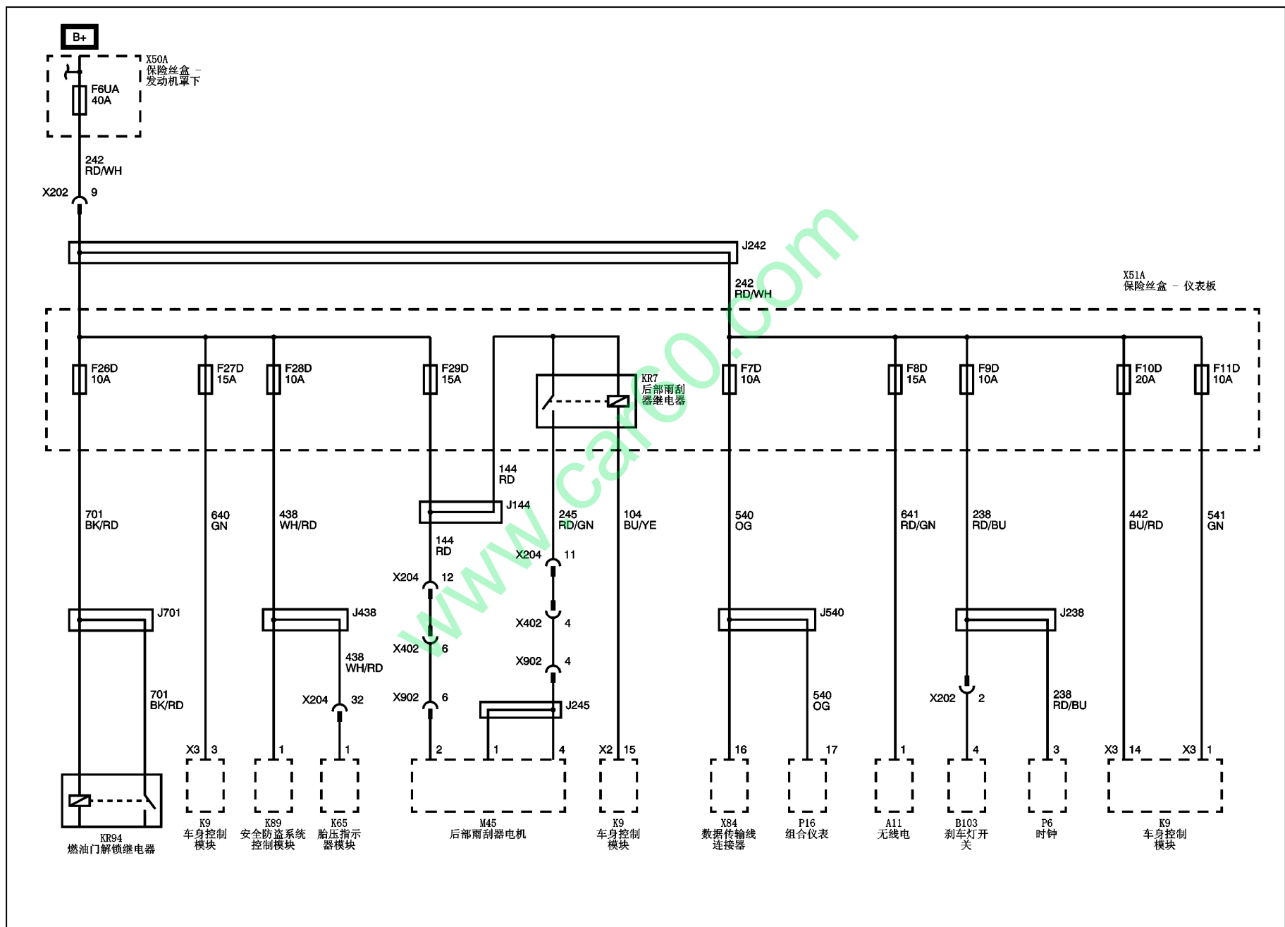
电源分布示意图 (F6UA, F7D, F8D, F9D, F10D, F11D, F26D, F27D, F28D, F29D 保险丝)
