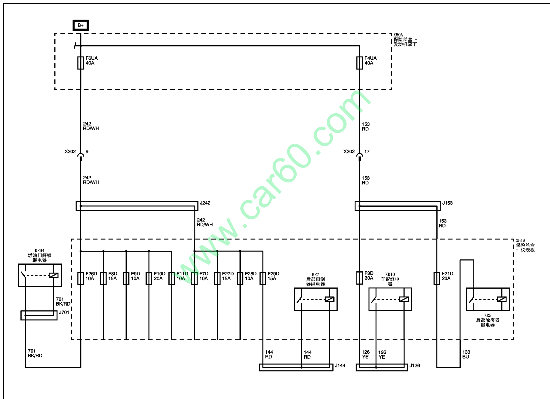
仪表板下保险盒电源分布
