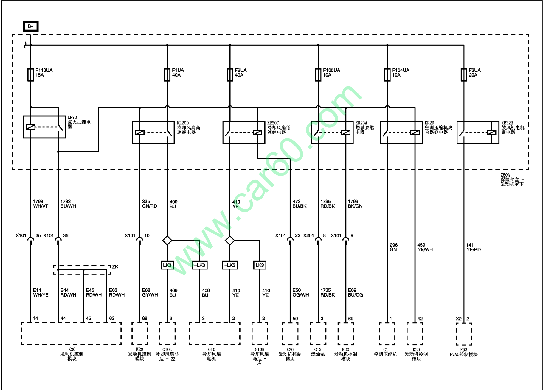
电源分布示意图 (F1UA, F2UA, F3UA, F104UA, F105UA, F110UA 保险丝)
