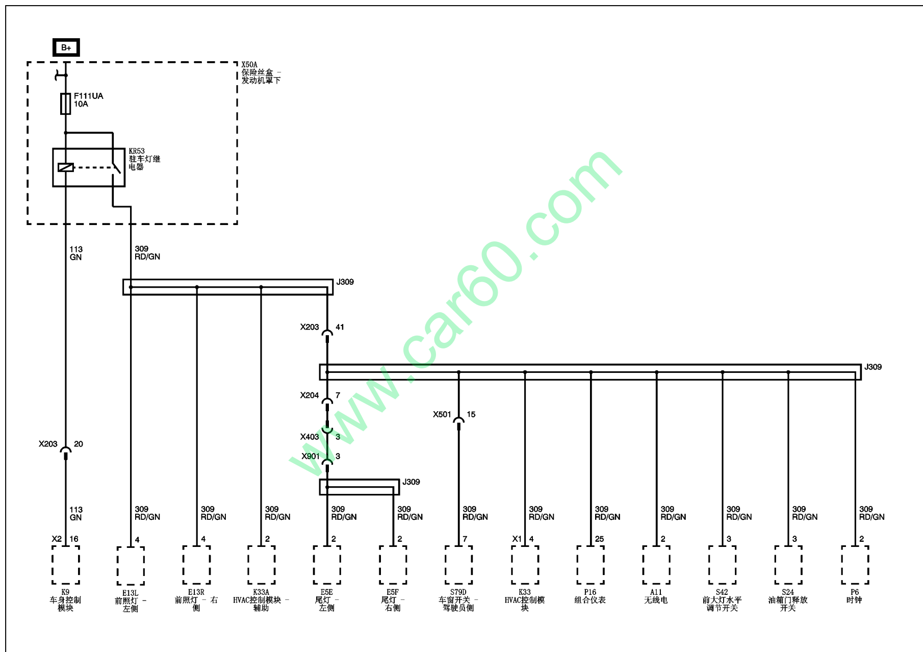
电源分布示意图 (F111UA 保险丝)
