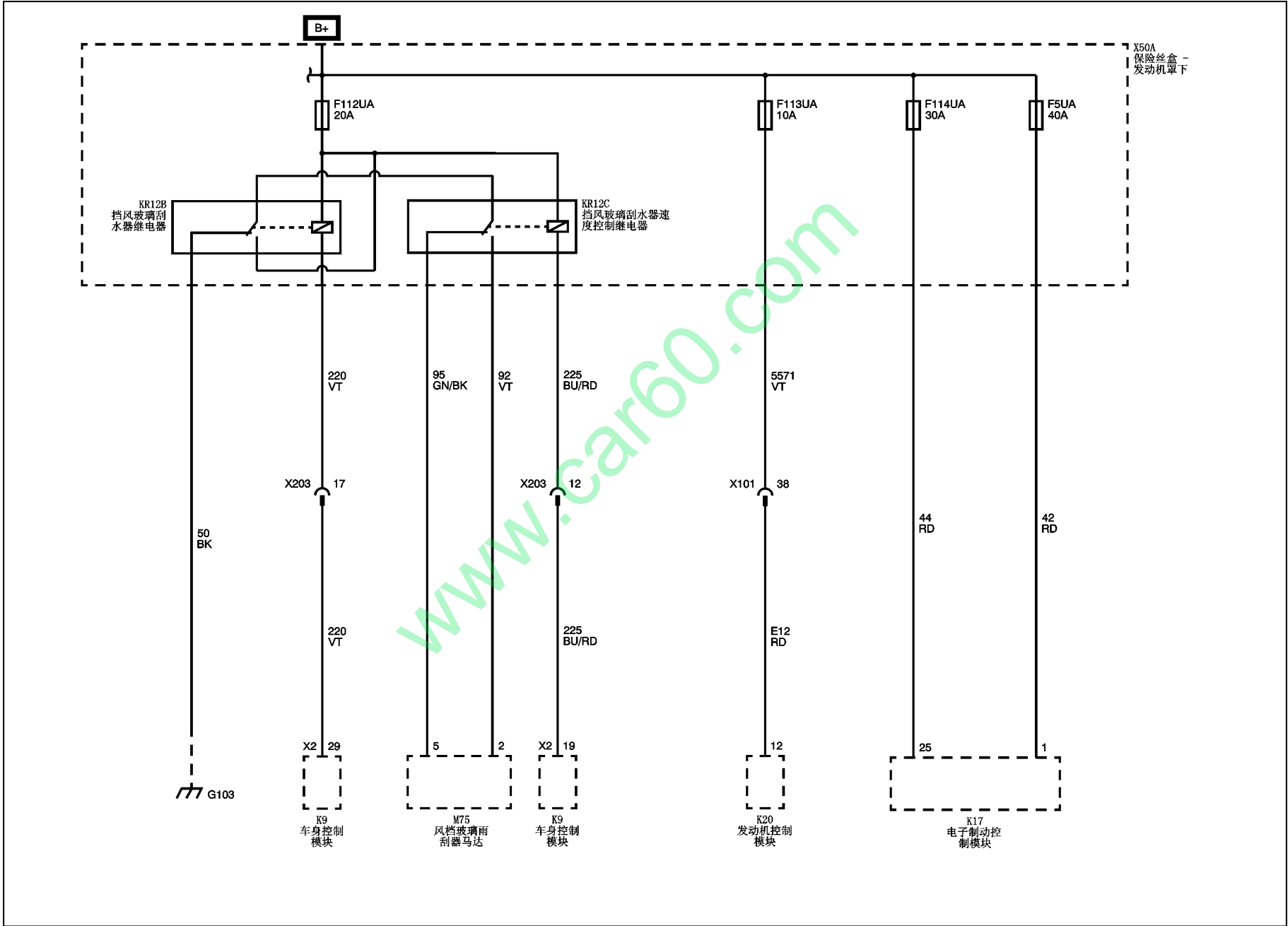
电源分布示意图 (F5UA, F112UA, F113UA, F114UA 保险丝)
